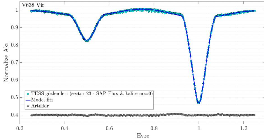
Şekil 10. V638 Vir sisteminin ışık eğrisi analizi sonucu elde edilen teorik model fiti ve çözümünden elde edilen artıklar
