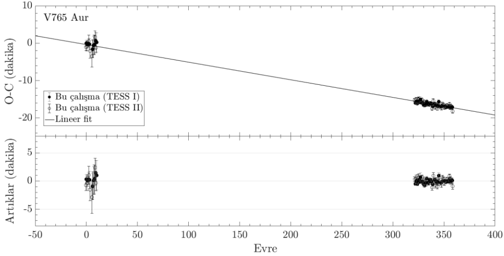
Şekil 3. V765 Aur sisteminin TESS gözlemlerinden okunan minimum zamanları kullanılarak oluşturulan O-C diyagramı. İçi dolu ve boş noktalar, sırasıyla, minimum I ve minimum II zamanlarını belirtmektedir. Siyah düz çizgi, O-C verisine yapılan lineer fiti göstermektedir. O-C verilerinden lineer fit çıkartılarak elde edilen O-C artıkları alt panelde gösterilmiştir.
